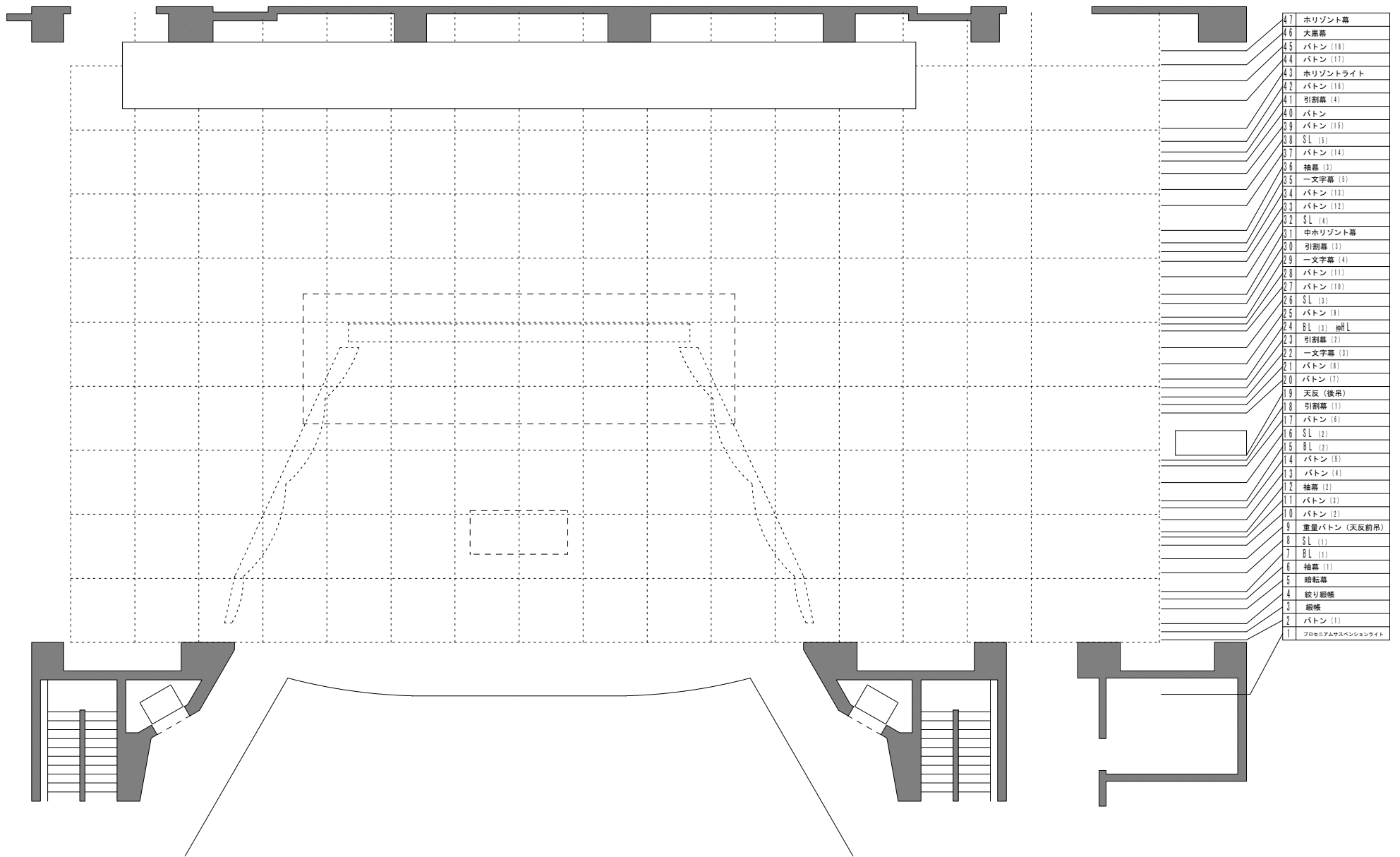
佐賀市文化会館 中ホール舞台平面図
