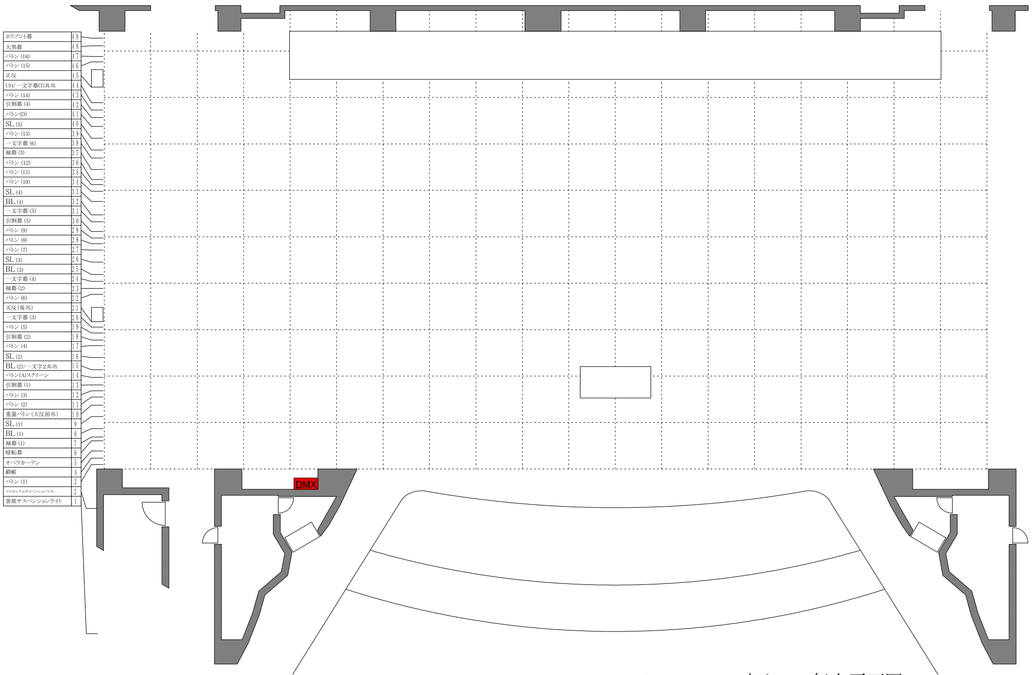
佐賀市文化会館 大ホール舞台平面図 1/150
