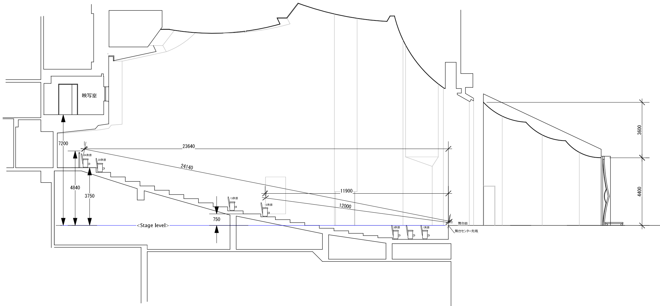
佐賀市文化会館 中ホール (センター部分) 断面図
