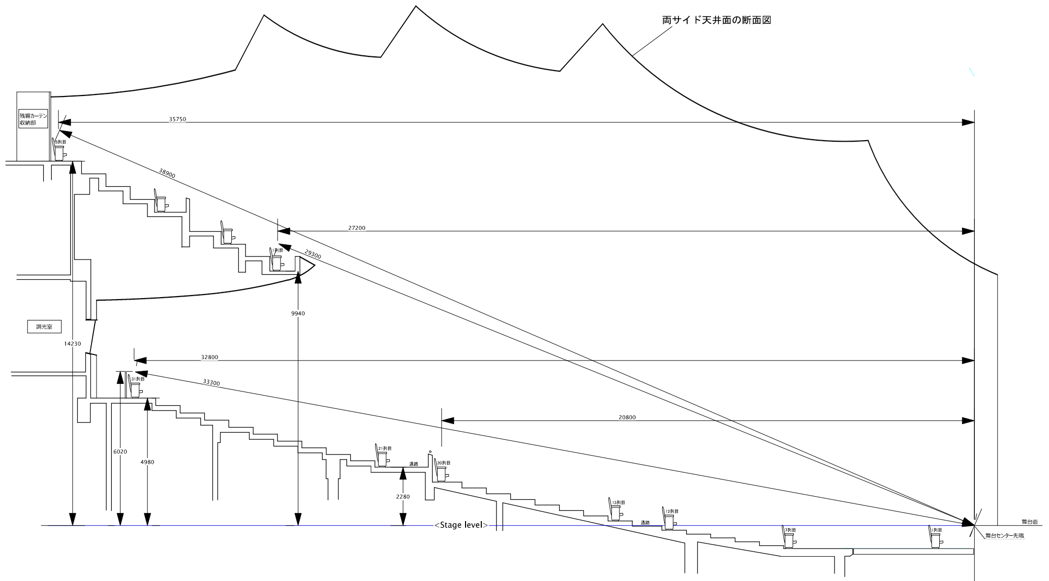
佐賀市文化会館 大ホール (センター部分) 断面図
