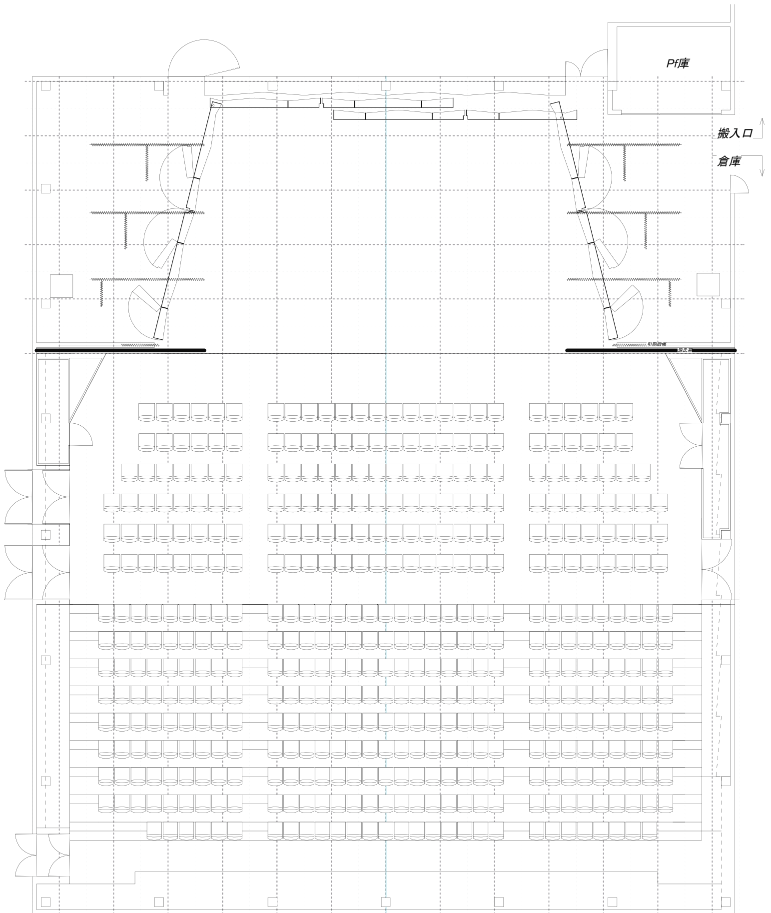
嬉野市社会文化会館 ホール平面図 1/125
