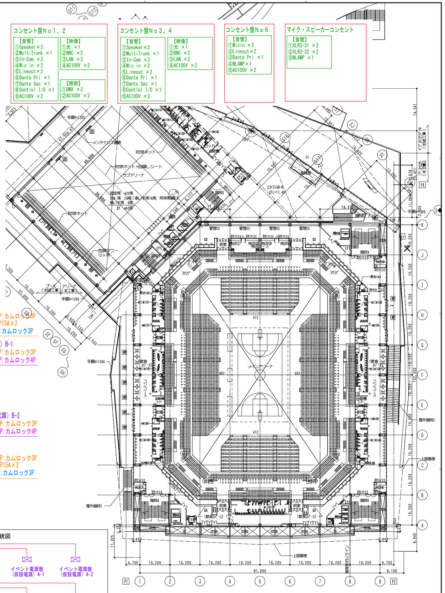
2階平面図
