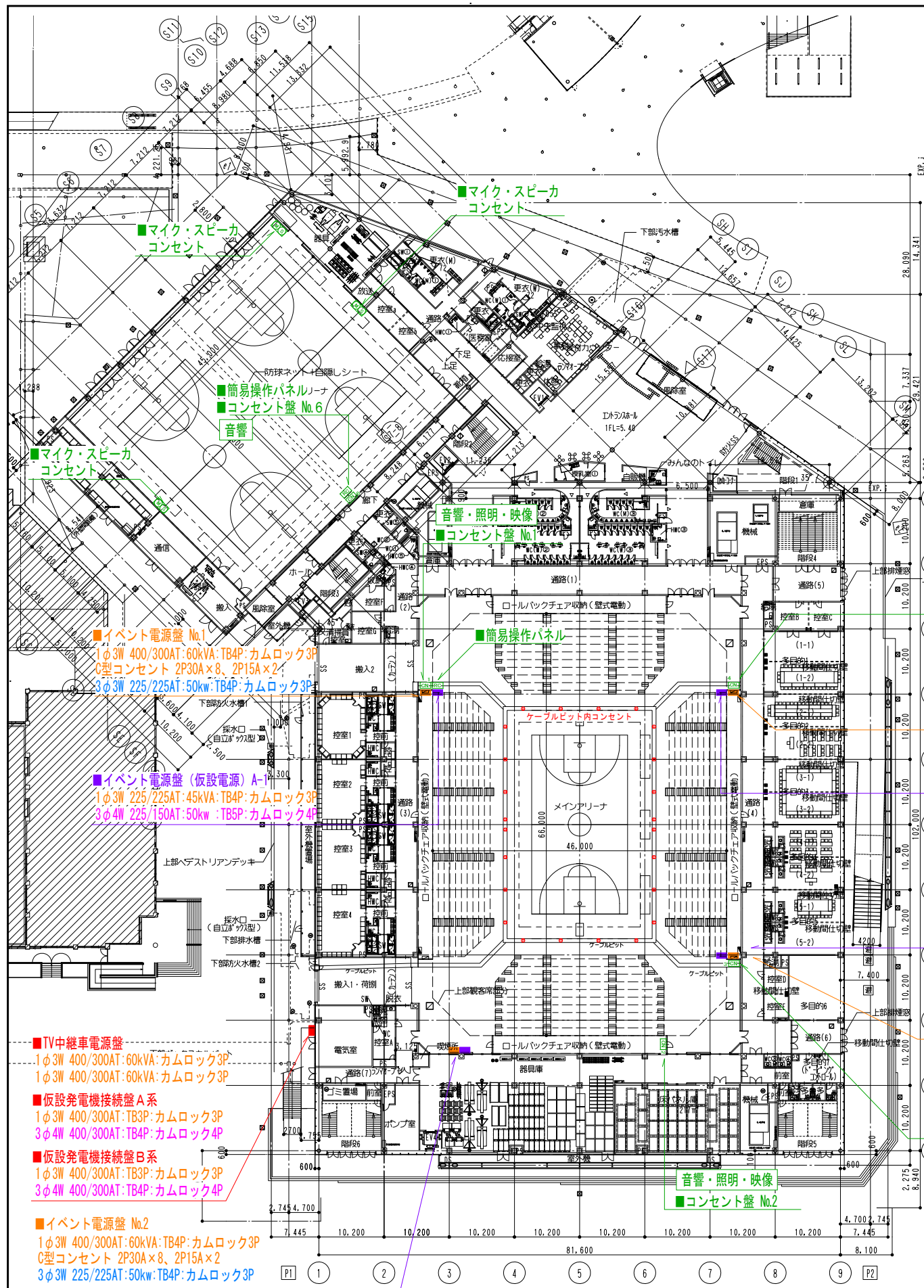
1階平面図
