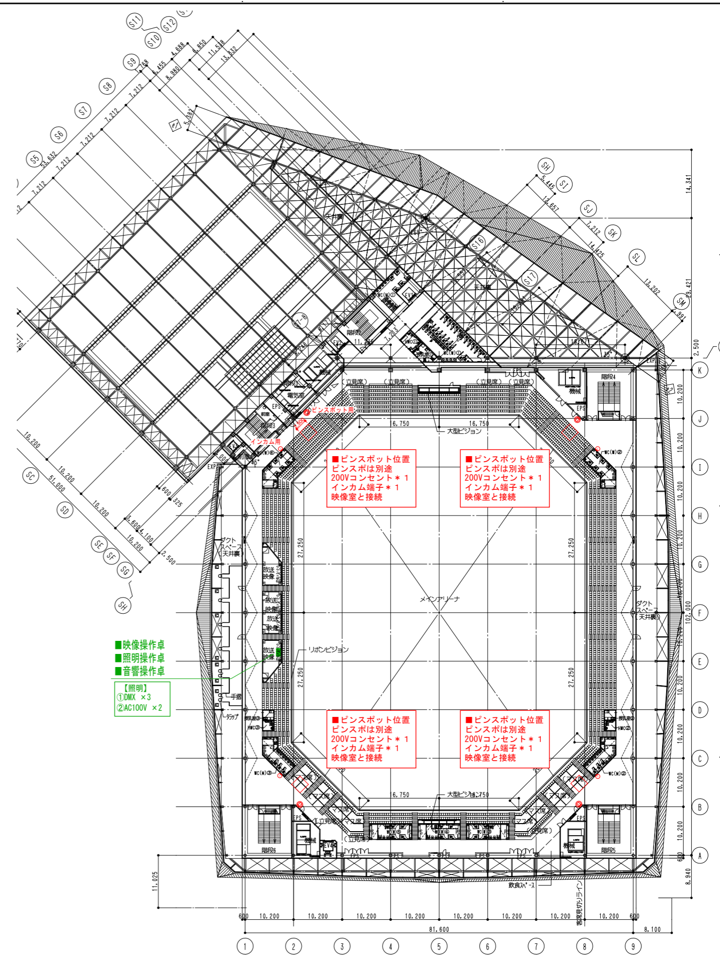
4階平面図
