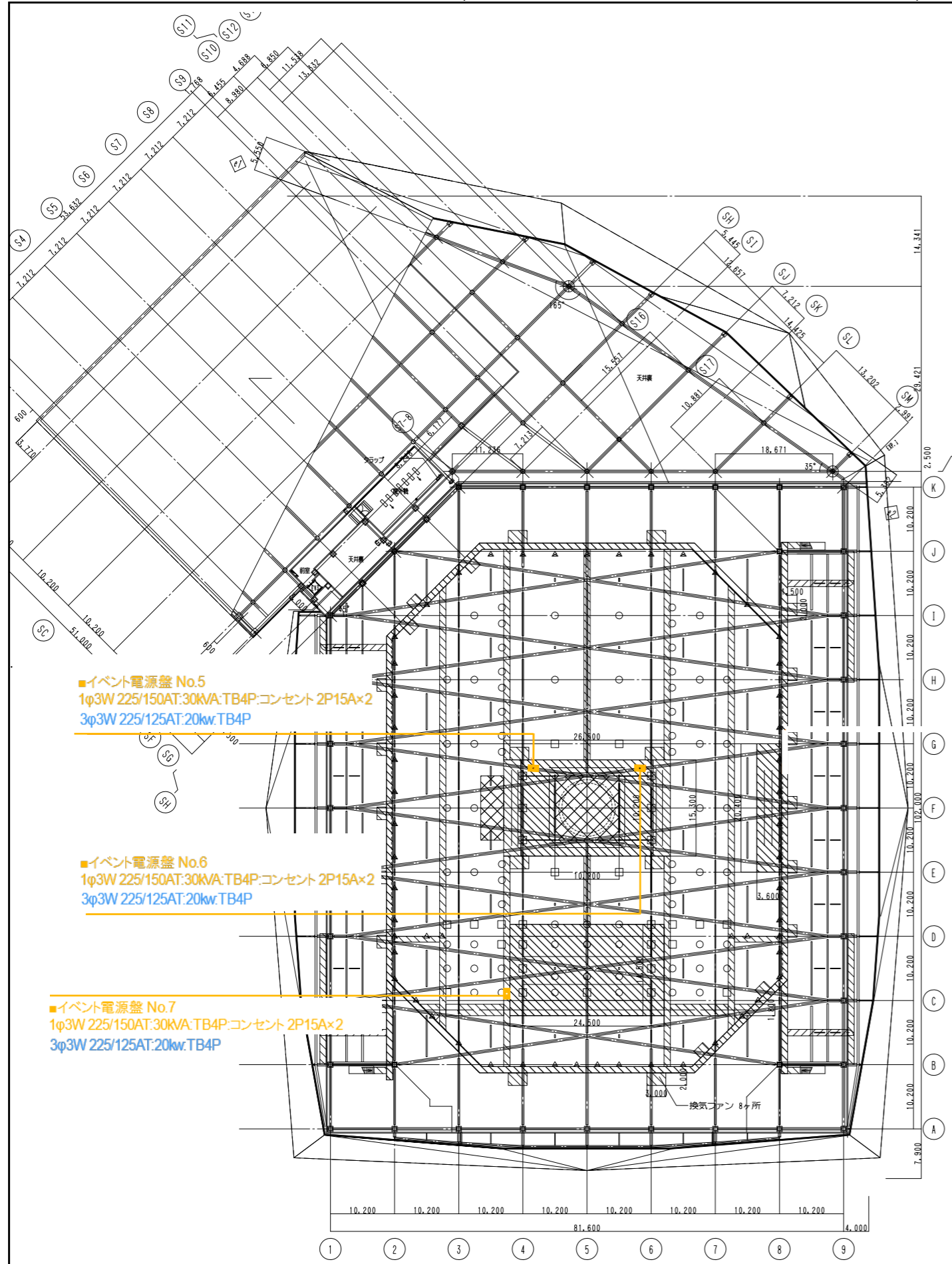
CW階平面図
