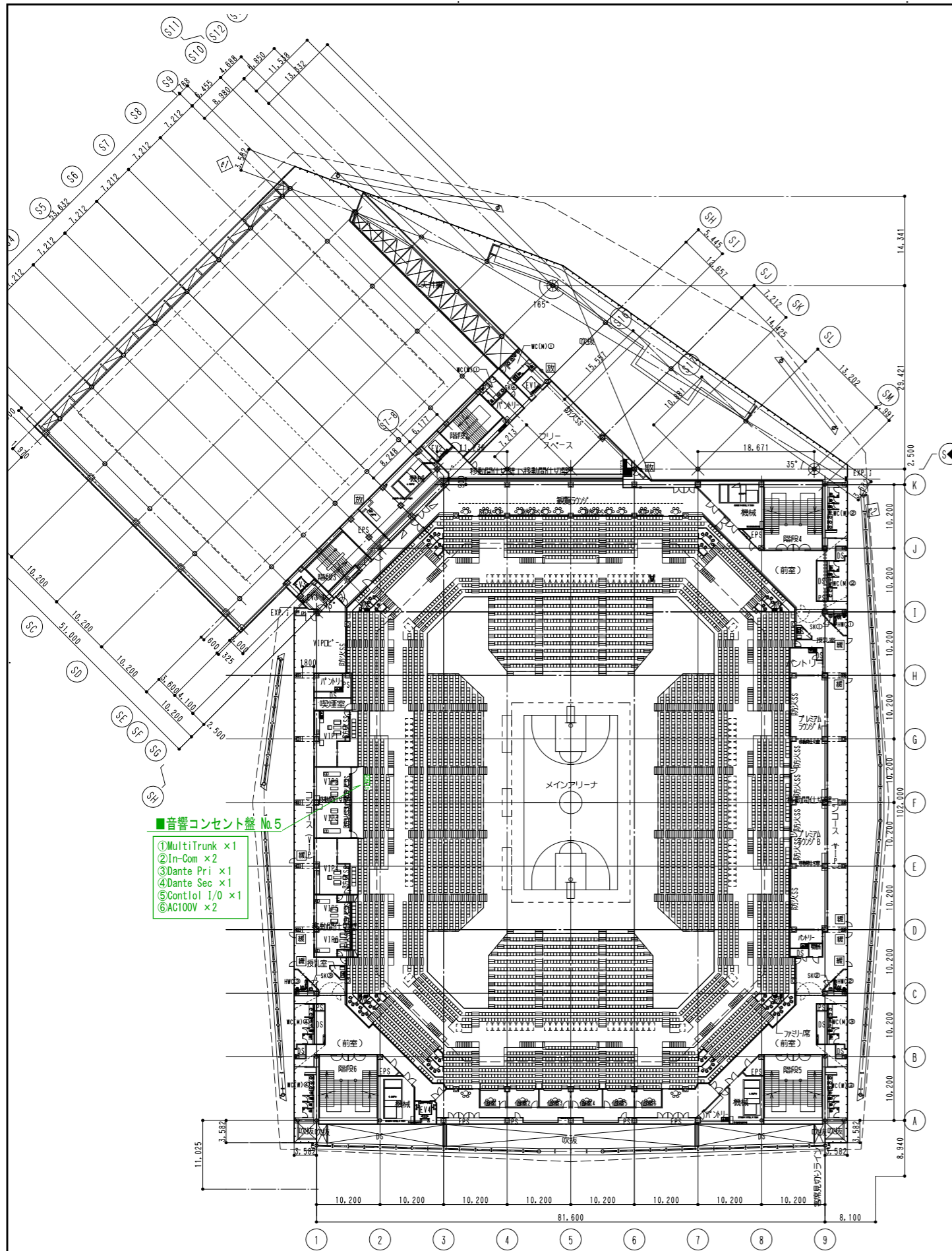
3階平面図
